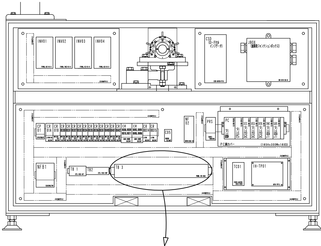
T B 3 端子台
